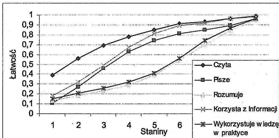
Rysunek 1. Krzywe charakterystyczne sprawdzanych umiejętności w zależności od wyniku w skali standardowej dziewiątki
