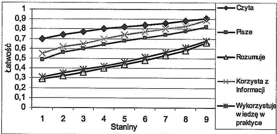
Rysunek 5. Krzywe charakterystyczne umiejętności w szkołach według wyniku w skali standardowej dziewiątki
